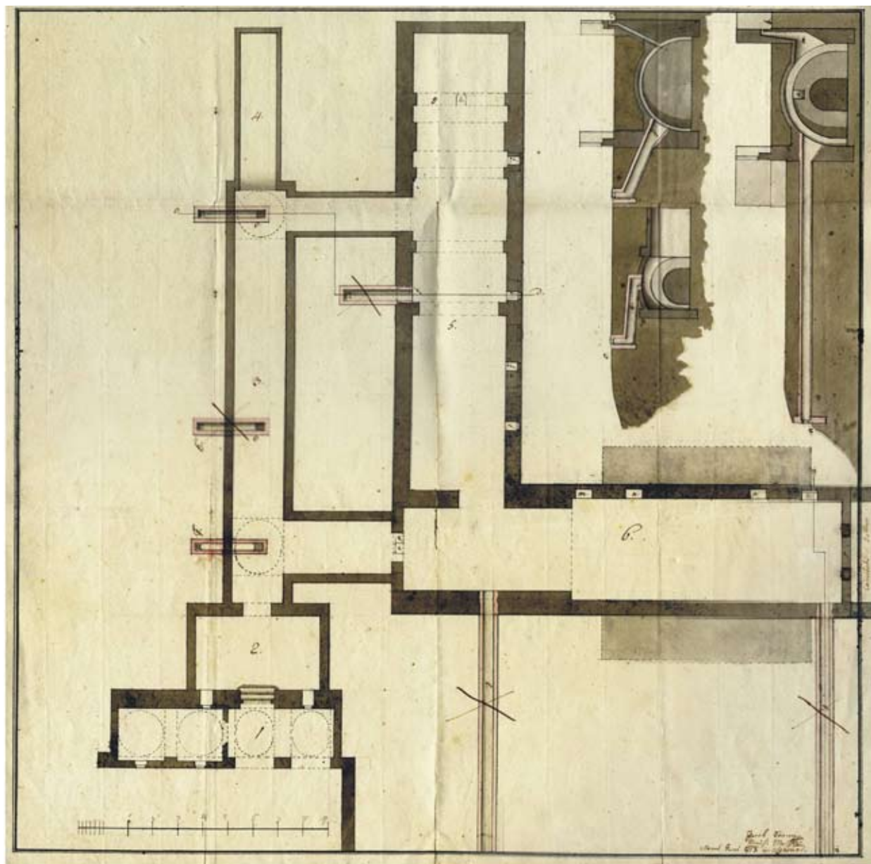
17. Jacob Stramm 1813-as terve a pince szellőzőrendszeréhez
