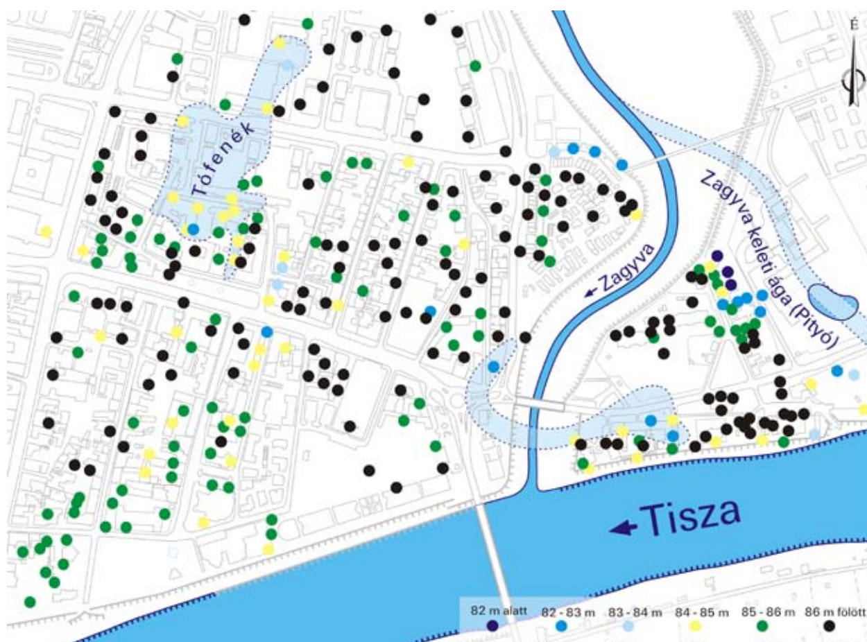
7. ábra. A történeti városmag területén leemélyített talajmechanikai fúrások, valamint az egykori folyómedrek és vízenyős, vízjárta területek elhelyezkedése – a pontok színezése a bolygatlan talajszintek Balti-tengerszint feletti magasságát mutatja (Kertész – Bana 2010, 68.)
