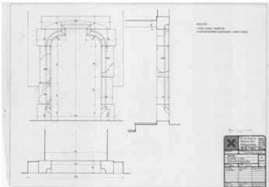
108. Fellekvár, keleti palota (J), a földszinti bejárat (Szerk. Kat.: 439/2.) rekonstrukciós terve Schönerné Pusztai Ilona–Erő Zoltán, 1986
