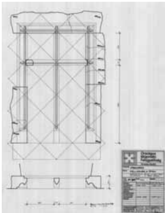
106. Fellegvár, ablak és ajtókeret elméleti rekonstrukciós rajza, Schönerné Pusztai Ilona, 1983
