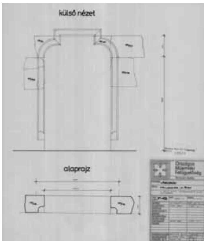
103. Fellegvár, nyugati palota (B), a földszinti bejárat (Szerk. Kat.: 439/5.) rekonstrukciós terve, Schönerne Pusztai Ilona–Máthé Géza, 1982
