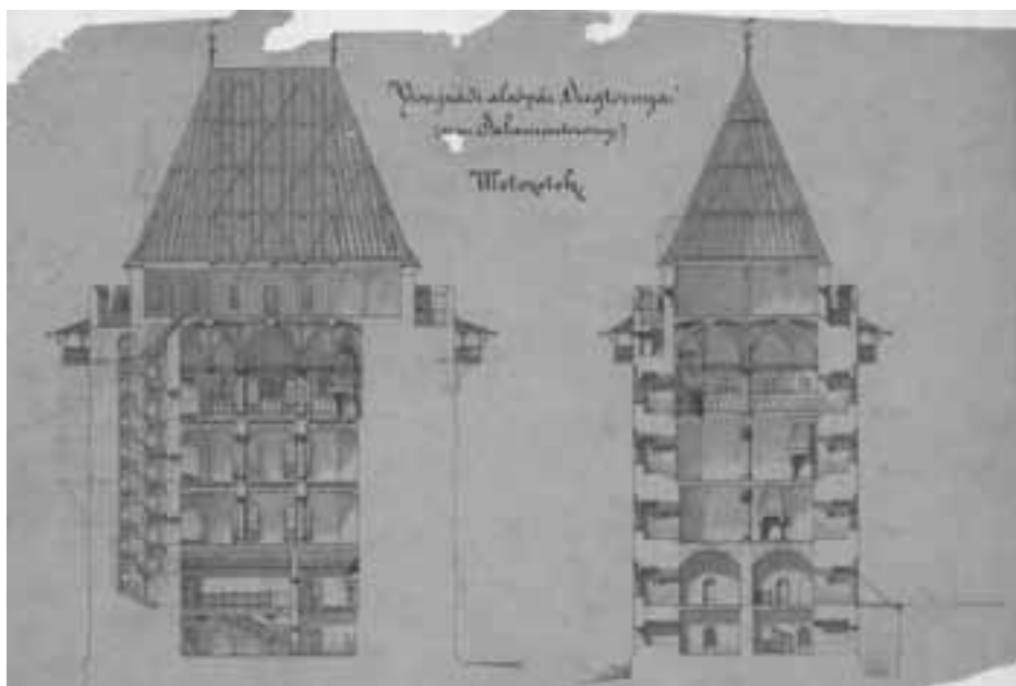
85. Salamon-torony, Schulek Frigyes helyreállítási terve, 1873
