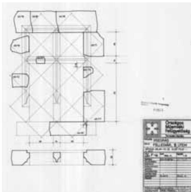
110. Fellegvár, keleti palota (J), első emeleti ablak (Szerk. Kat.: 439/3.) rekonstrukciós terve, Schönerné Pusztai Ilona, 1984
