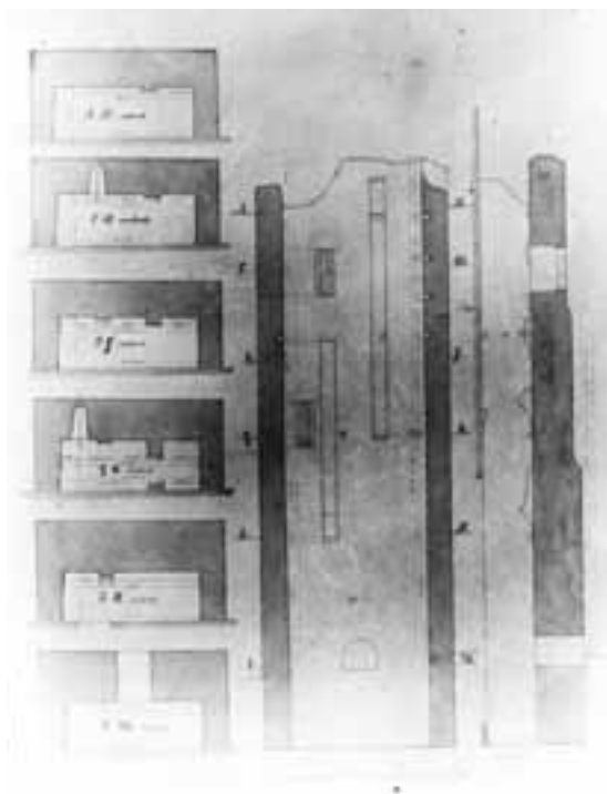
53. A Salamon-torony nyugati fióktornyának felmérési rajza, Zsigmondy Gusztáv, 1872(?)
