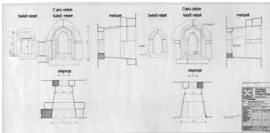
102. Fellegvár, a nyugati palota (B) udvari homlokzati ablakainak kiegészítési terve, Schönerne Pusztai Ilona–Máthé Géza, 1982
