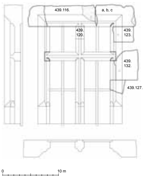
168.b. Fellegvár, ablakkeret elméleti rekonstrukciós rajza, Bozóki Lajos, 1993. Szerk. Kat.: 439/8.
