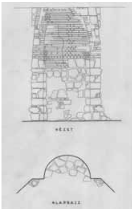
45. A Salamon-torony harmadik emeleti kandallójának felmérési rajza, Sedlmayr János, 1960
