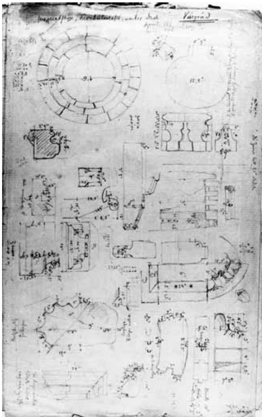
128. A Fellegvár napvilágra került kőfaragványai, Henszlmann Imre felmérési rajza, 1880 körül
