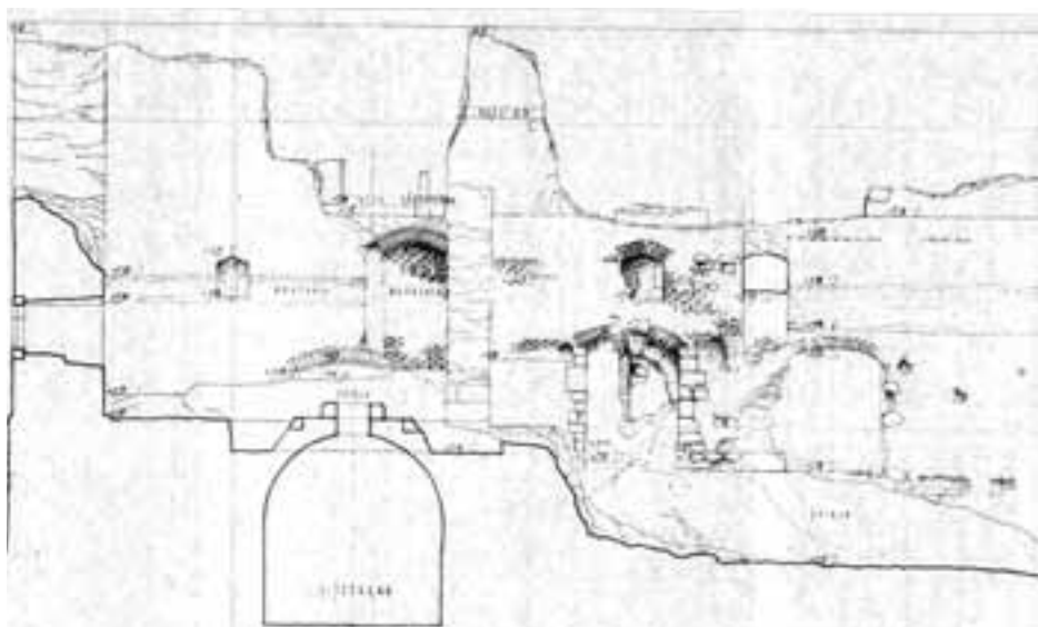
17. Fellegvár, az északnyugati palota (E) déli fala, belső nézet; felmérési rajz, Schönerné Pusztai Ilona és munkatársai, 1985
