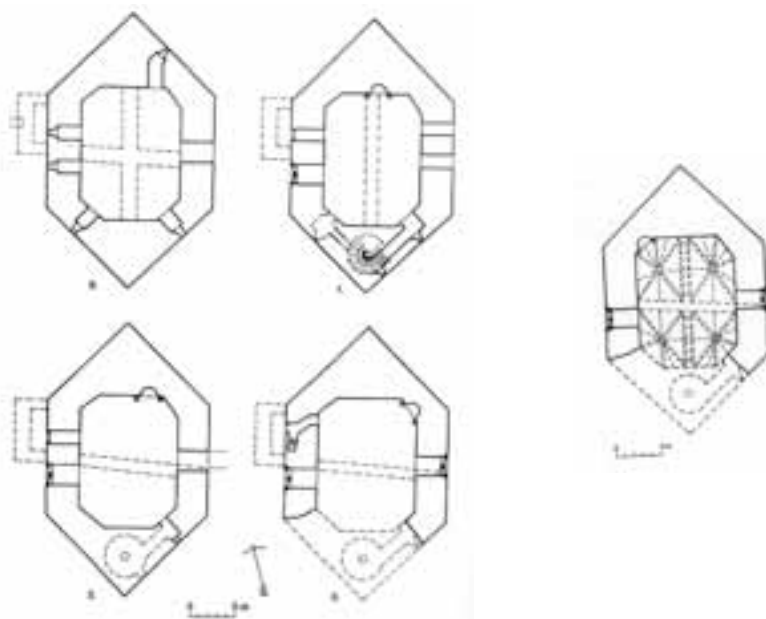
48. A Salamon-torony szintenkénti alaprajza a feltételezett keresztfalakkal és boltozattal, Bozóki Lajos
