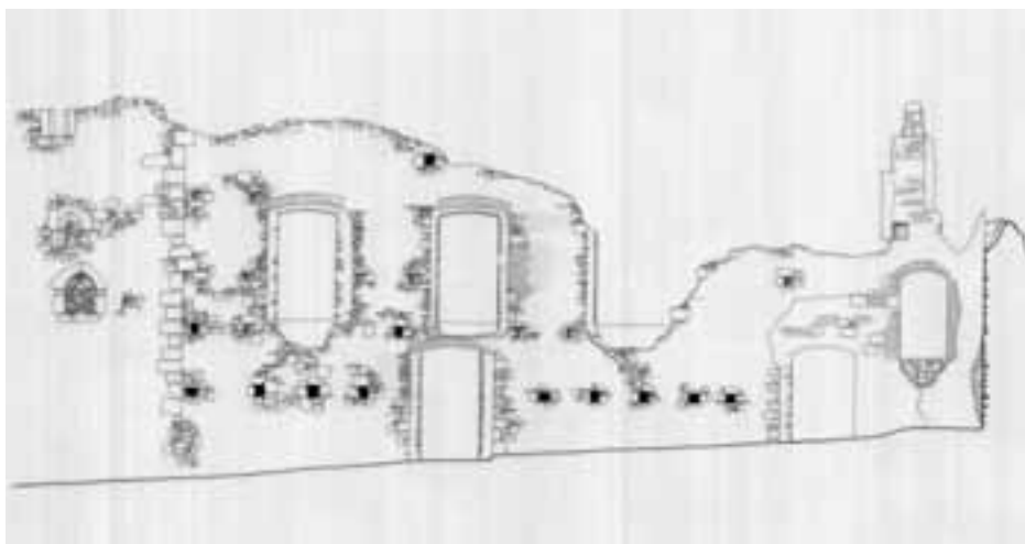
12. Fellegvár, a nyugati palota (B) mellé északról beépített palota (C) és az északi lépcsőház (D) udvari homlokzata helyreállítás előtt; felmérési rajz, Schönerné Pusztai Ilona és munkatársai, 1978
