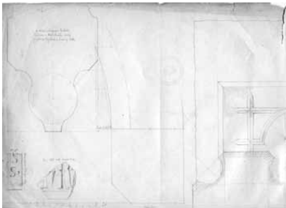
133. A Fellegvár napvilágra került kőfaragványai és leletei, Henszlmann Imre felmérési rajza, 1880 körül
