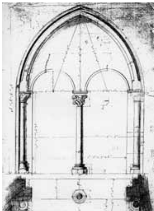
38. Salamon-torony, keleti homlokzat, a negyedik emeleti ablak a középoszlop 1930-ban kiváltott fejezetével, Gregus Antal felmérése, 1872
