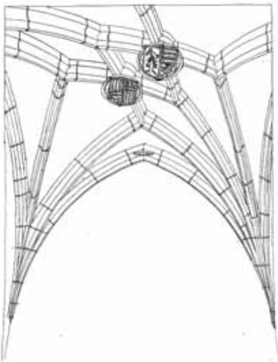
70. Fellegvár, a déli kaputorony (A) Mátyás- és Beatrix-címeres boltozata (Szerk. Kat.: 439/9.), Szőke Balázs rekonstrukciós rajza
