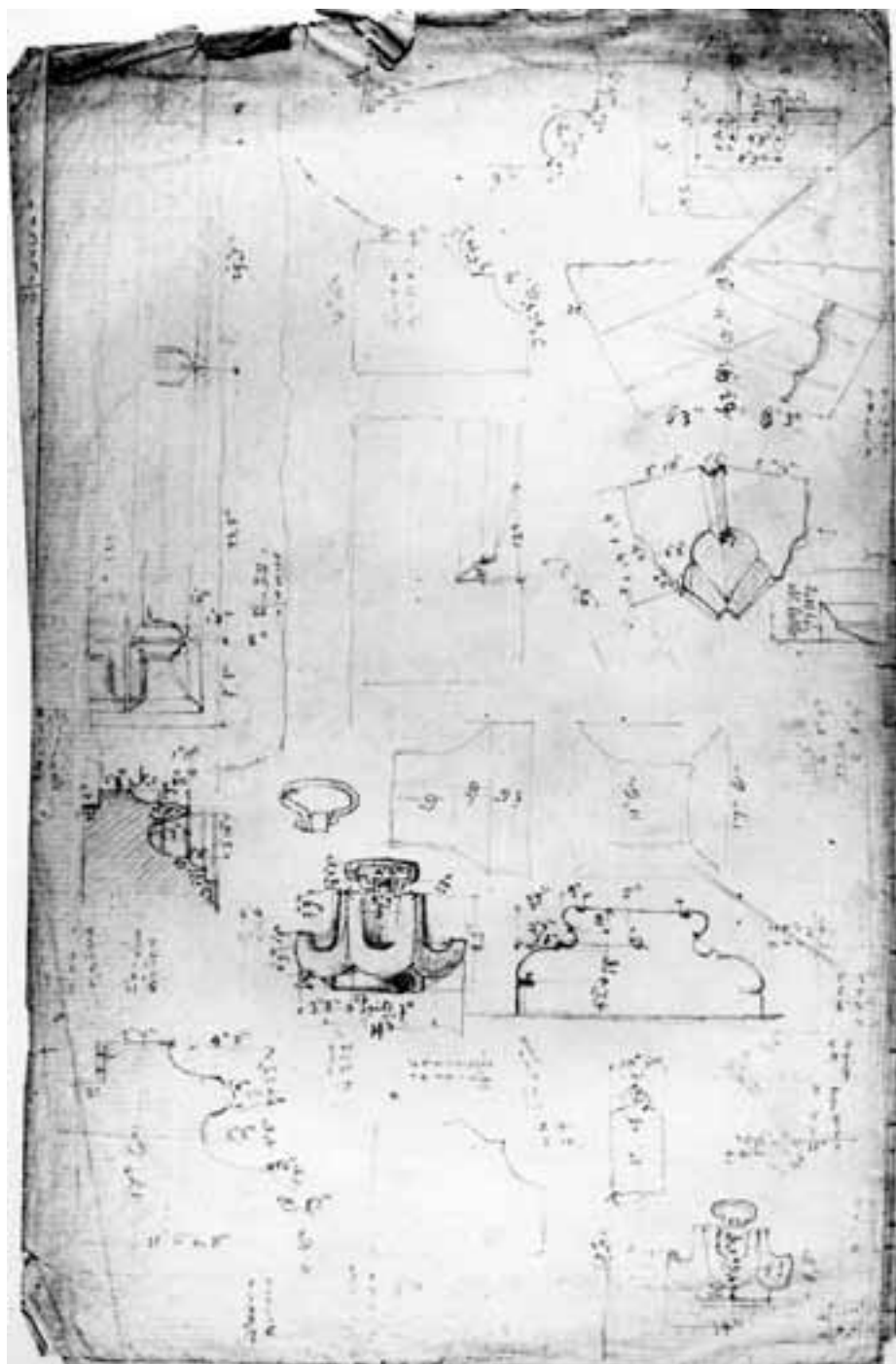
131. A Fellegvár napvilágra került kőfaragványai és leletei, Henszlmann Imre felmérési rajza, 1880 körül
