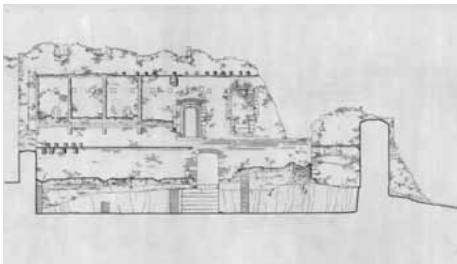
11. Fellegvár, a nyugati palota (B) keleti falának belső nézete helyreállítás előtt; felmérési rajz, Schönerné Pusztai Ilona és munkatársai, 1976
