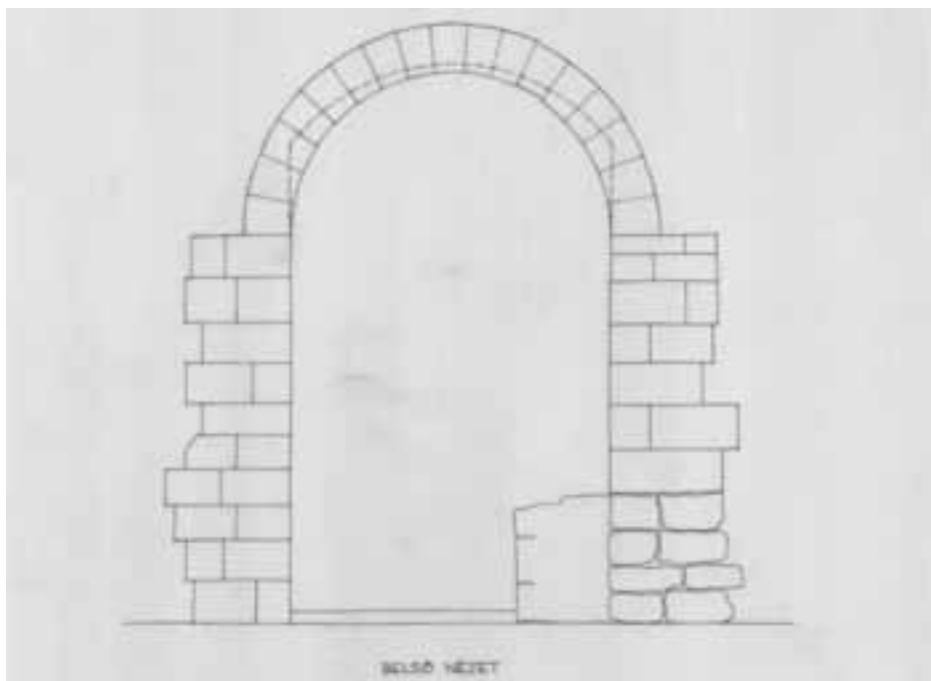
49. Salamon-torony, a második emelet keleti, ajtóvá alakított ikerablakának fülkéje, jobb oldalon a lábazati zónában az egykori keresztfal megmaradt csonkjja; felmérési rajz, Sedlmayr János, 1959
