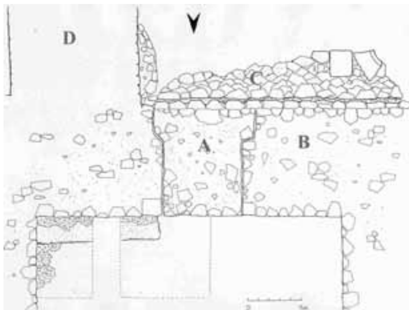
114. A keleti torony déli fala kutatás után: „A” befalazott ajtó, „B” a torony déli fala, „C” köpenyezés a torony déli fala előtt, „D” keleti várfal; Bozóki Lajos felmérési rajza, 1997
