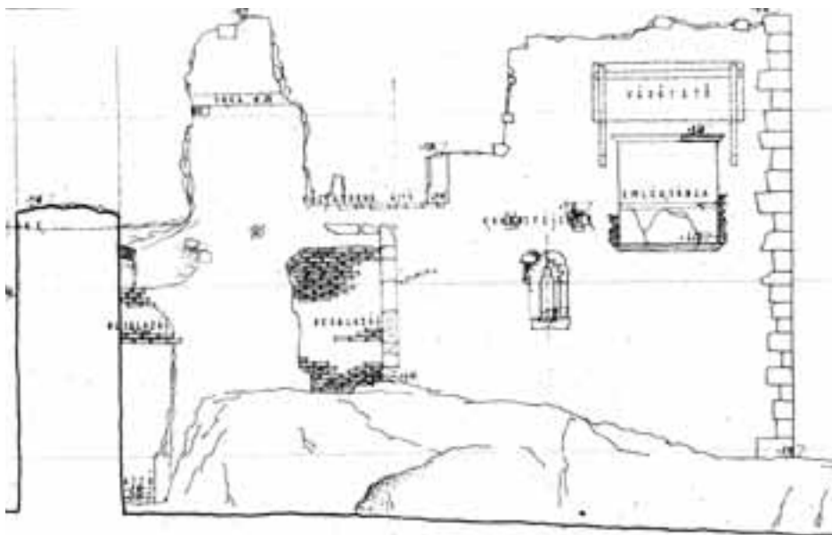
16. Fellegvár, az északnyugati palota (E) udvari homlokzata, a koronaöri emléktábla (Szerk. Kat.: 439/10.) maradványaival; felmérési rajz, Schönerné Pusztai Ilona és munkatársai, 1985
