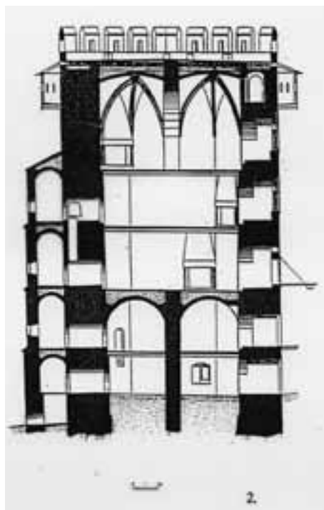
56. A Salamon-torony a 14. században, kelet-nyugat irányú metszet, Buzás Gergely rajza
