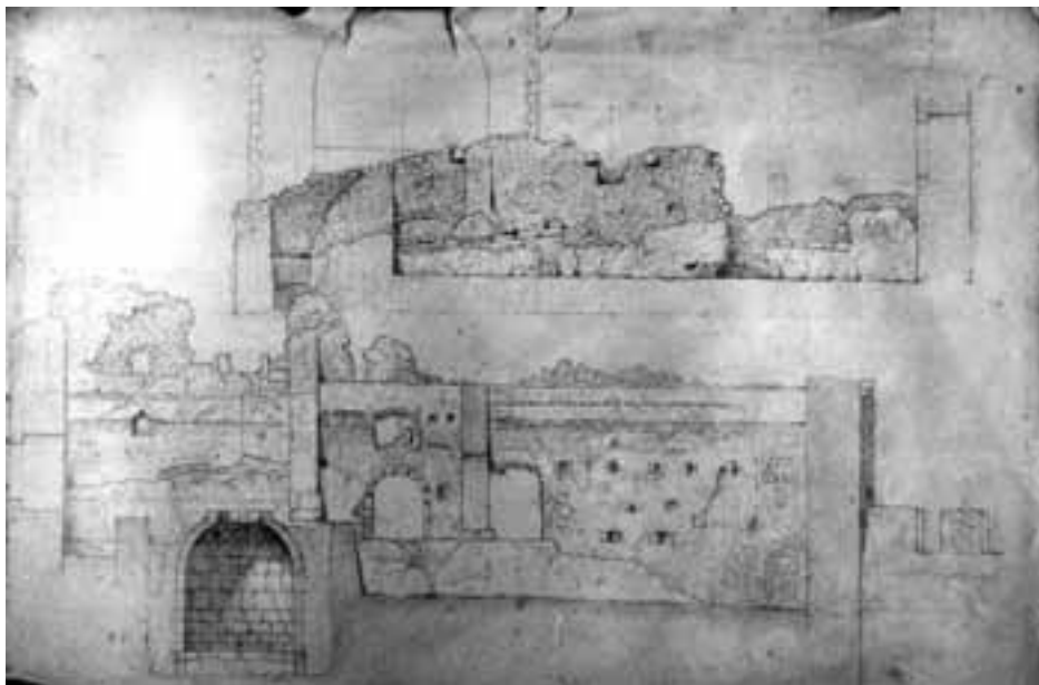
124. Fellegvár, Henszlmann Imre vagy Zsigmondy Gusztáv felmérési rajza, 1880 körül; fent az északkeleti palota (F) belső déli fala, lent az északnyugati palota (E) belső, déli fala
