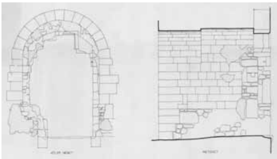
37. Salamon-torony, keleti homlokzat, a második emelet bejáratát alakított ikerablakának felmérési rajza, Sedlmayr János, 1960
