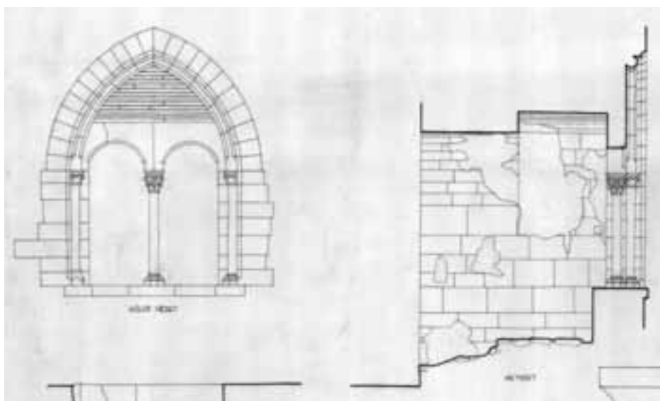
41. Salamon-torony, keleti homlokzat, a negyedik emeleti ablak felmérési rajza, Sedlmayr János, 1960
