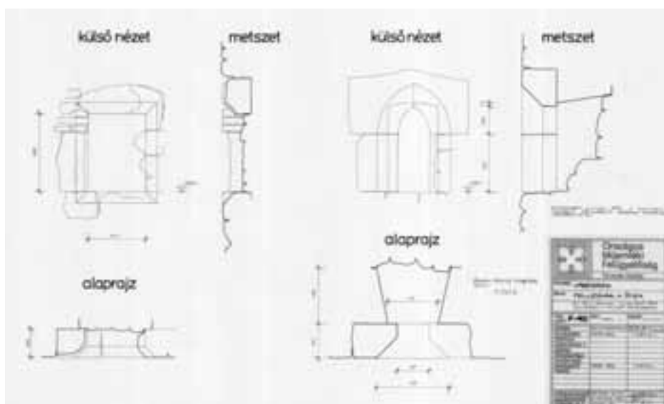
101. Fellegvár, a nyugati palota (B) udvari homlokzati ablakainak kiegészítési terve, Schönerné Pusztai Ilona-Máthé Géza, 1982
