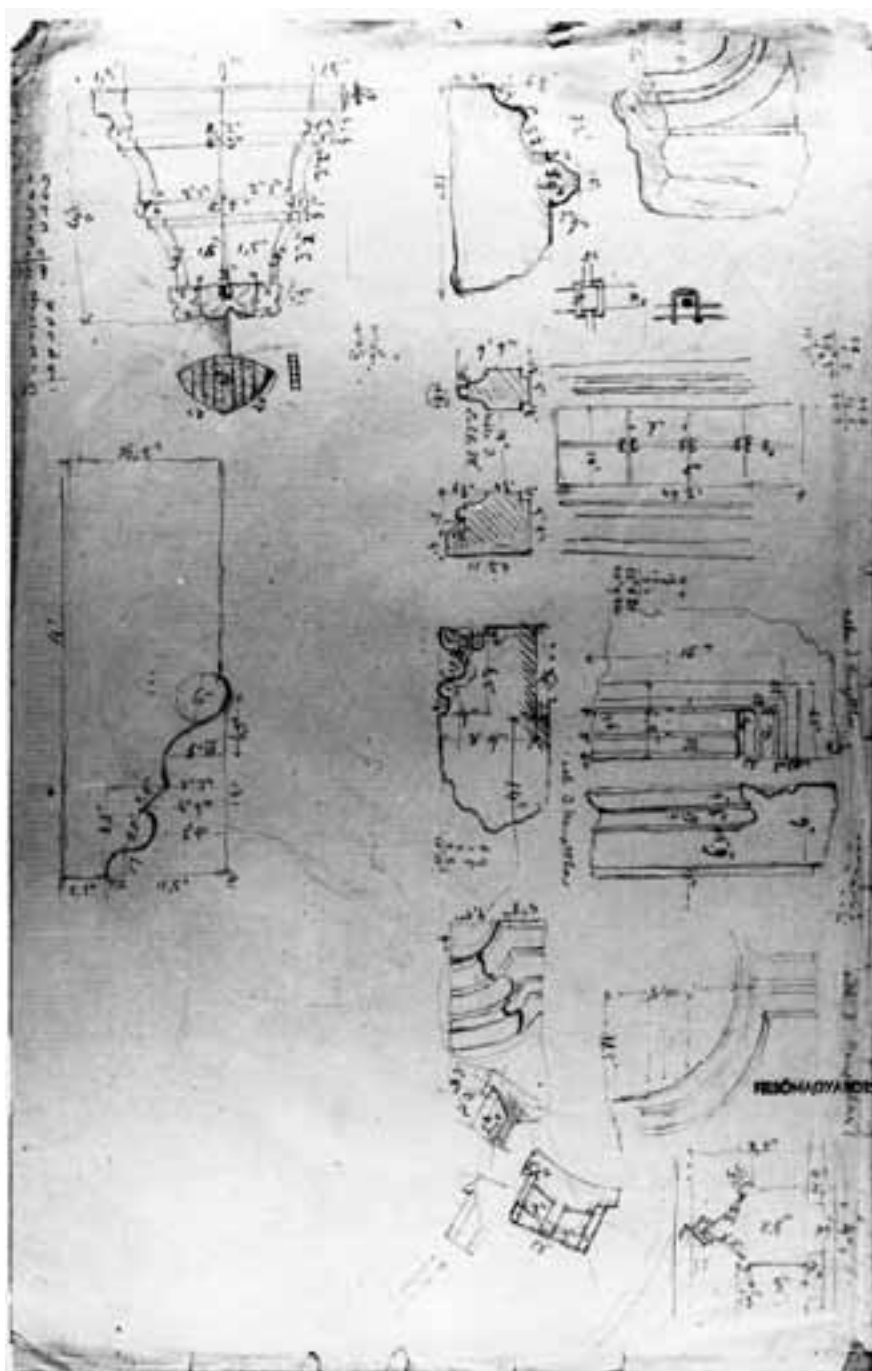
130. A Fellegvár napvilágra került kőfaragványai, jobbra fent talán a királyi palota kerengőjéhez tartozó konzol, Henszlmann Imre felmérési rajza, 1880 körül
