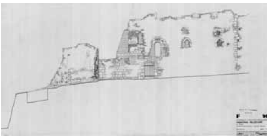
9. Fellegvár, a déli kaputorony (A) nyugati falának belső nézete és a nyugati palota (B) udvari homlokzata helyreállítás előtt; felmérési rajz, Schönerné Pusztai Ilona és munkatársai, 1976
