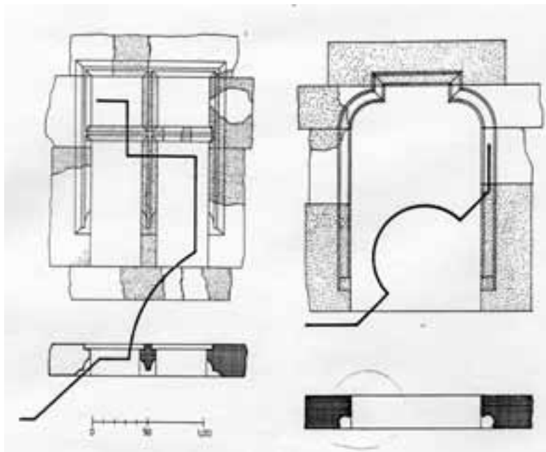
106. Fellegvár, ablak és ajtókeret elméleti rekonstrukciós rajza, Schönerné Pusztai Ilona, 1983
