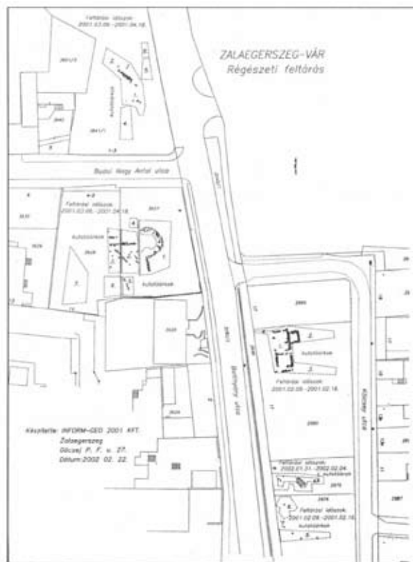
5. Az egerszegi vár ÉK-i külső bástyájának ásatási alaprajza (Vándor 2006 nyomán)
