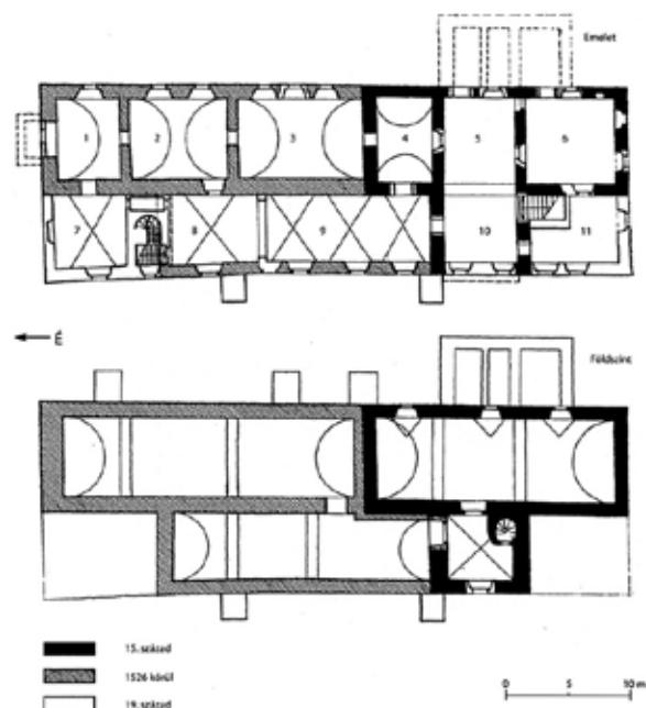
20. A devecseri kastély alaprajza (Koppány 2009 nyomán)
