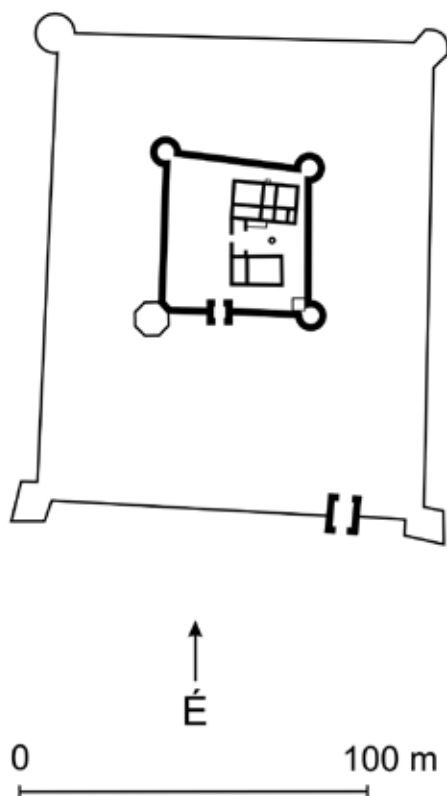
12. Az egerszegi vár 17. századi rekonstruált alaprajza
