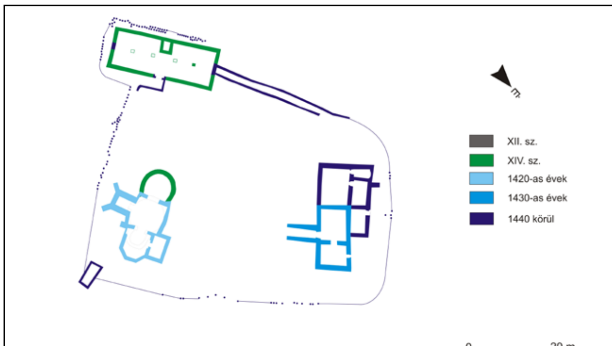
46. A kishánai kastély alaprajza 1440 körül
