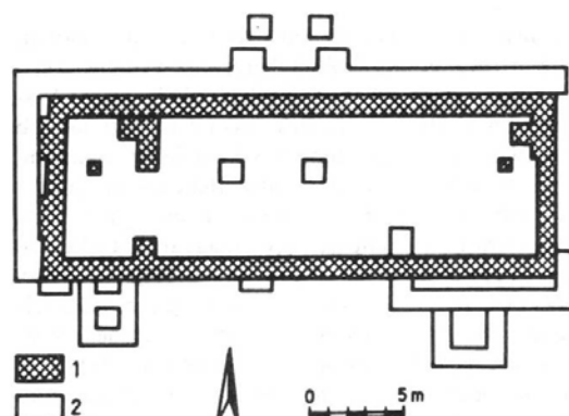
19. A XI-XII. századi belényesszentmiklósi hercegi udvarház alaprajza
