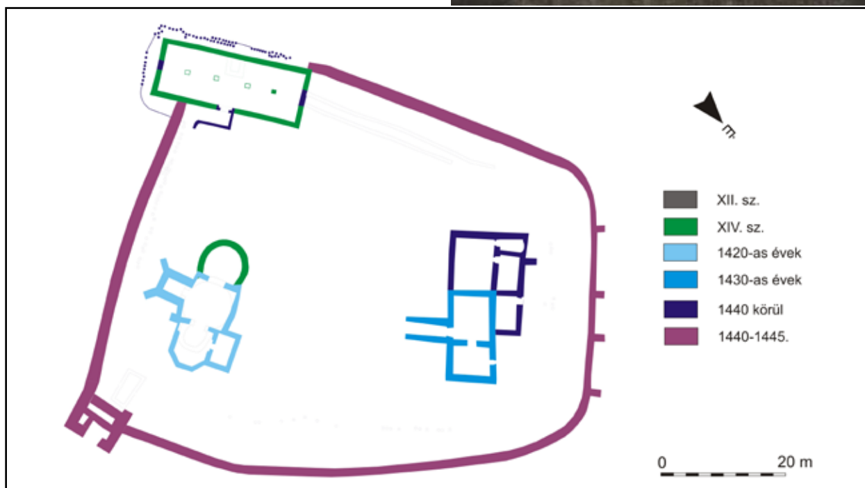
59. A kishánai vár alaprajza 1445-ben
