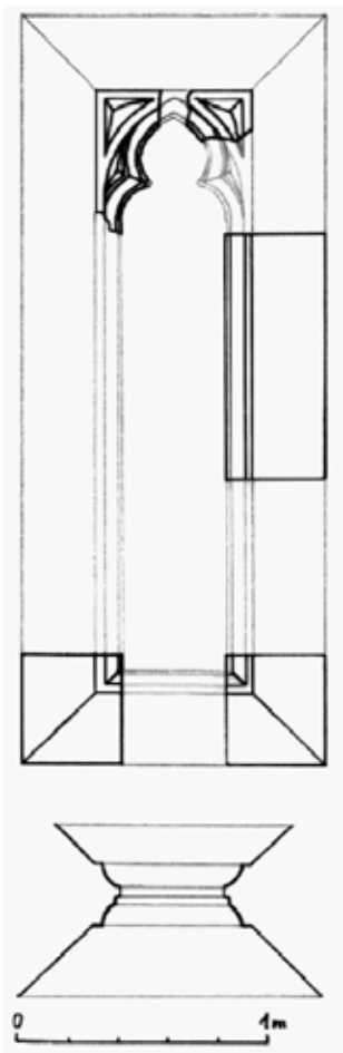
32. A kishánai templom szentélyablaka (Nagy Szabolcs Balázs rajza)
