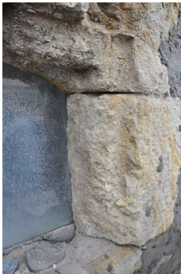
99. A belső katorony lépcsőházának ablakkerete
