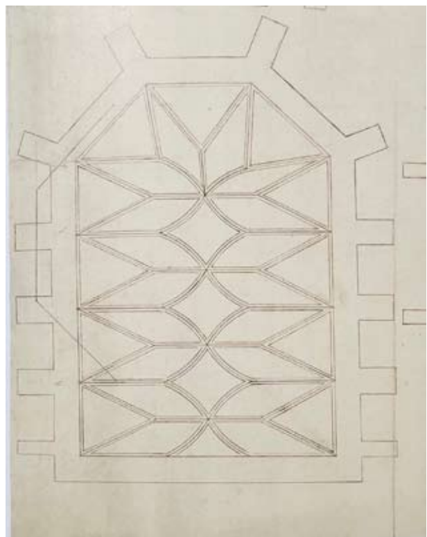
73. Szentélyboltozat alaprajza (16.877) a bécsi Stephanskirche építőpáholyának gyűjteményéből (BÖKER 2005 nyomán)
