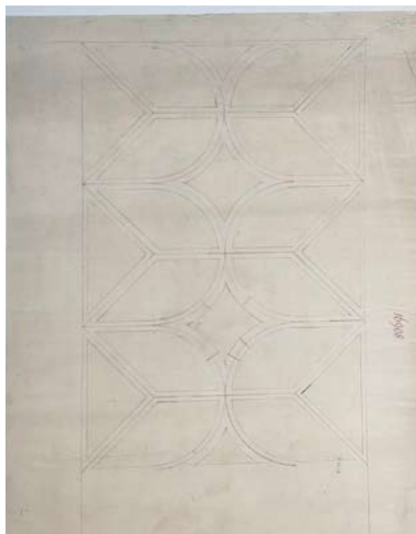
75. Boltozat alaprajza (16.908) a bécsi Stephanskirche építőpáholyának gyűjteményéből (BÖKER 2005 nyomán)
