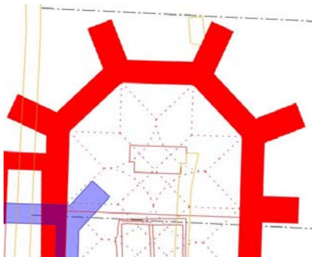
117. A visegrádi ferences templom főoltárnak alaprajza (rajz: Buzás Gergely)
