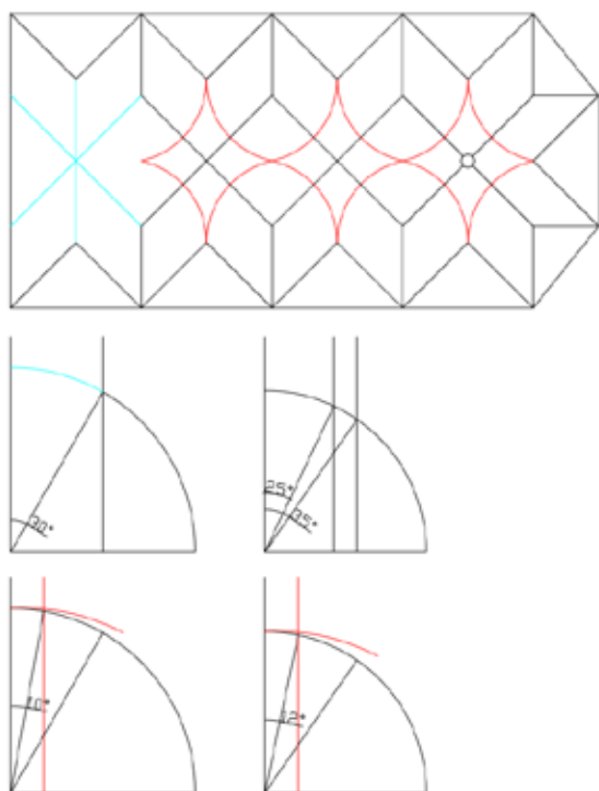
51. A visegrádi ferences templom szentélyboltozatának szerkesztése (rajz: Szőke Balázs)
