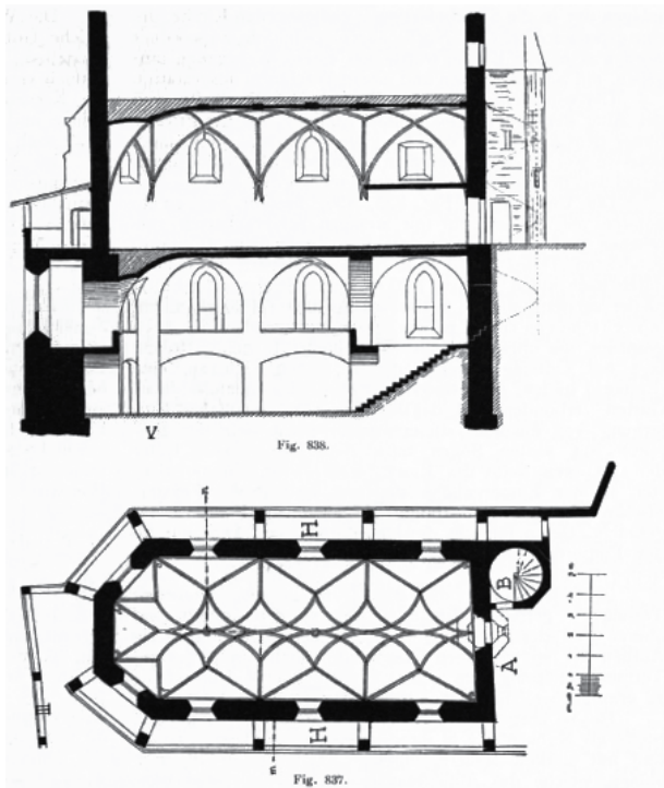
71. A znojmoi Szent Vencel-kápolna (Prokop 1904 nyomán)
